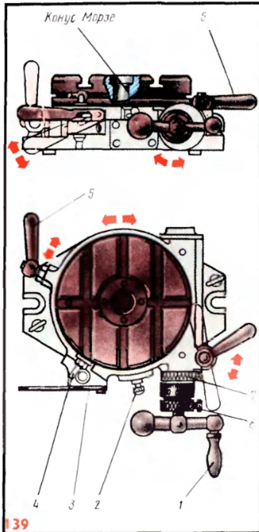
Круглый поворотный стол с ручным приводом
