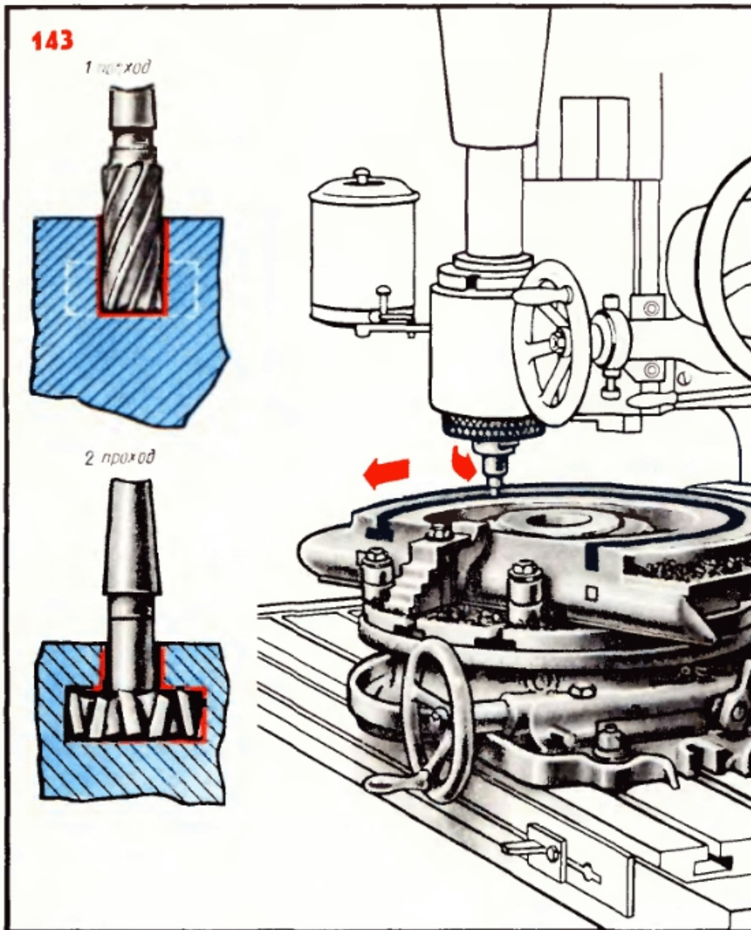
Фрезерование кругового Т-образного паза
