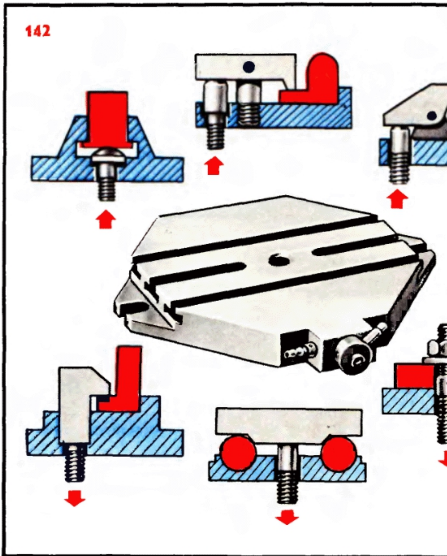
Схемы наладок для закрепления заготовок на столе с диафрагменным
