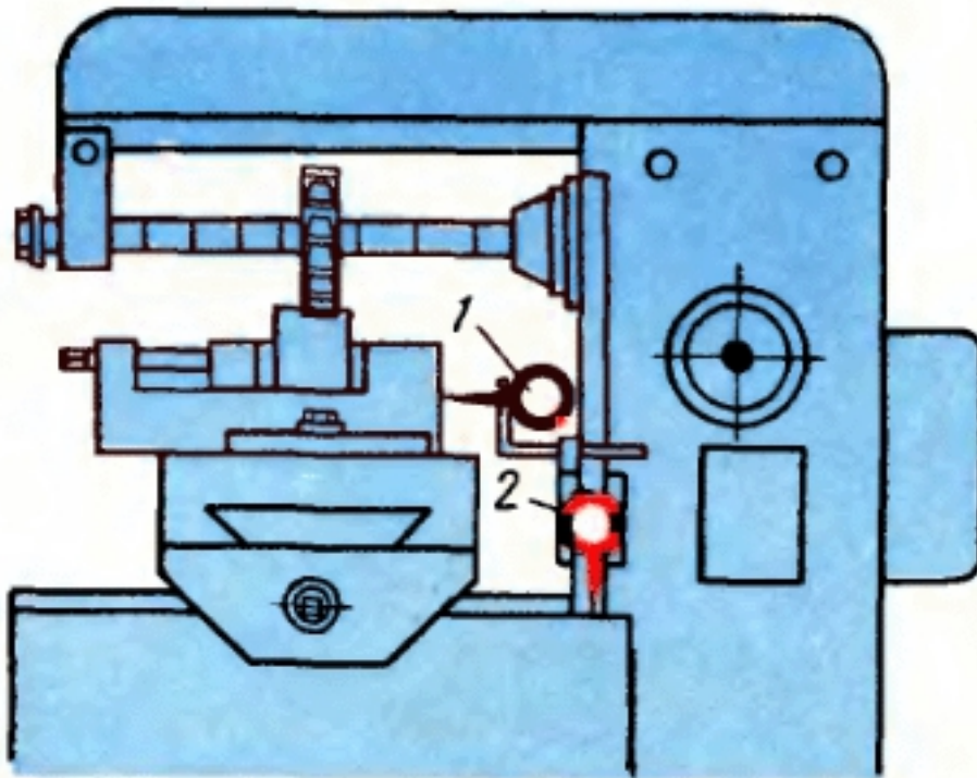
Схема расположения индикаторных упоров
