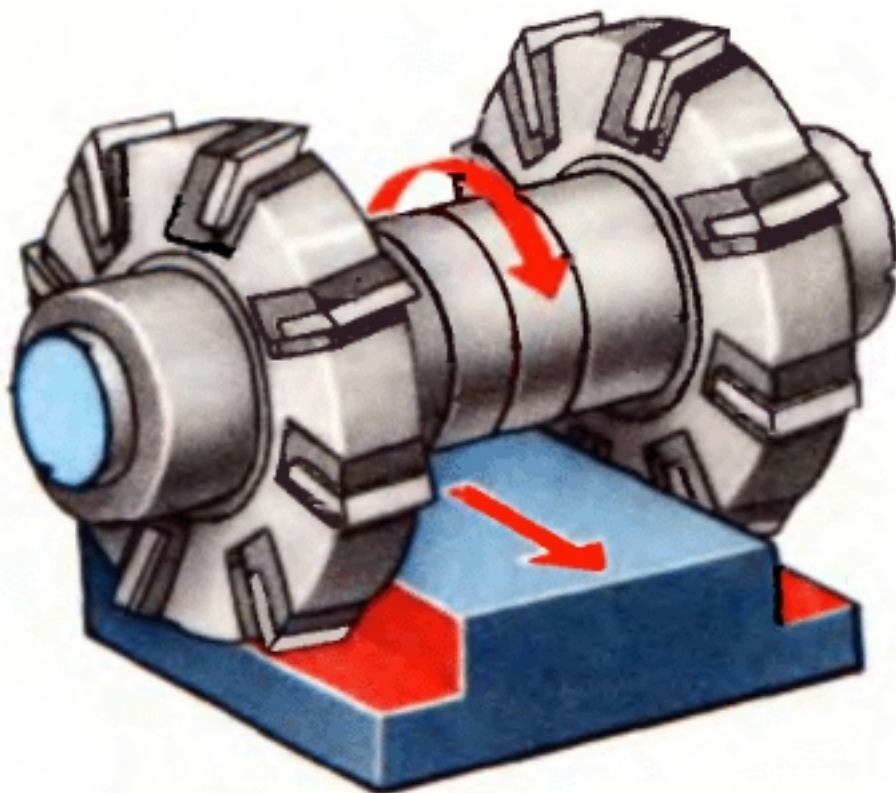
Фрезерование уступов набором фрез
