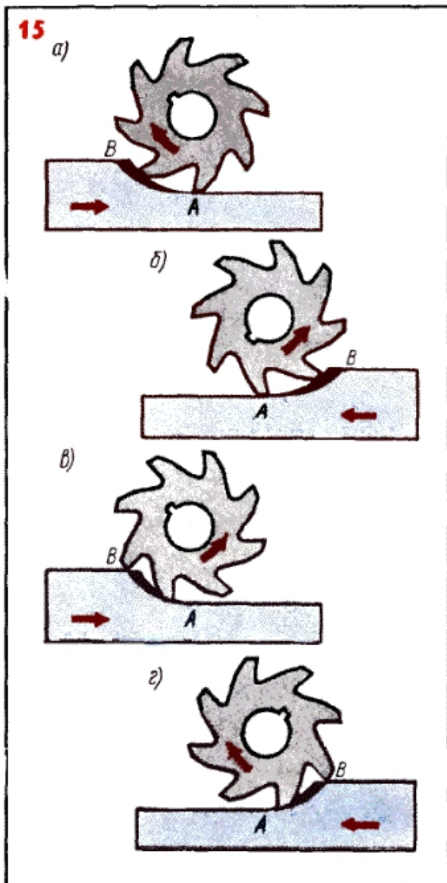
Схемы фрезерования
