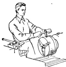
Рис 47 Свинчивание патрона при помощи ключа
