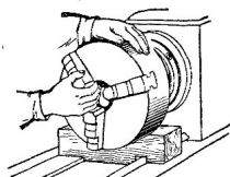
Рис 46 Навинчивание на шпиндель тяжелого патрона
