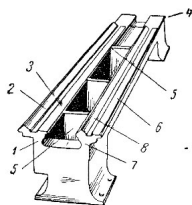
Рис. 2. Станина токарного станка
